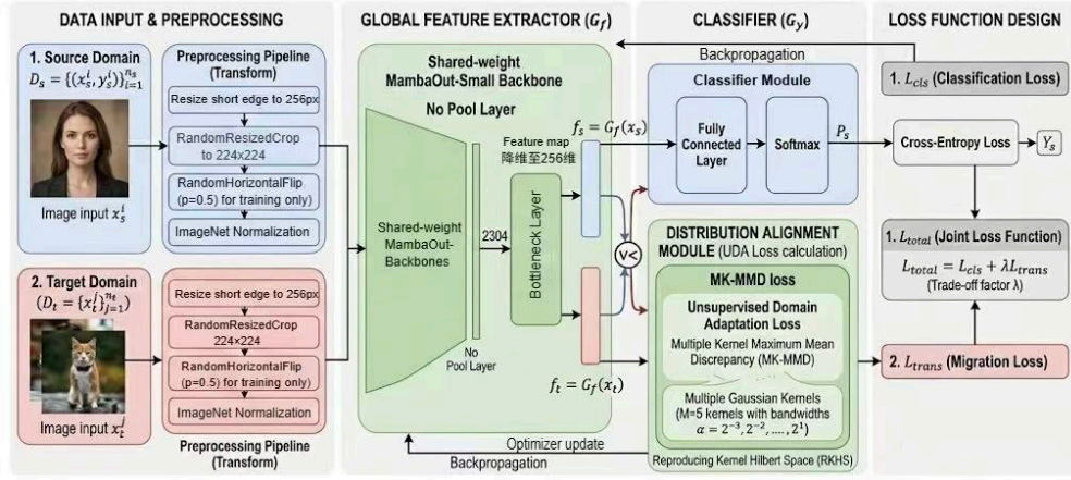
图 2.2: MambaOut-Small 去全局池化骨干与 MK-MMD 域自适应架构。
